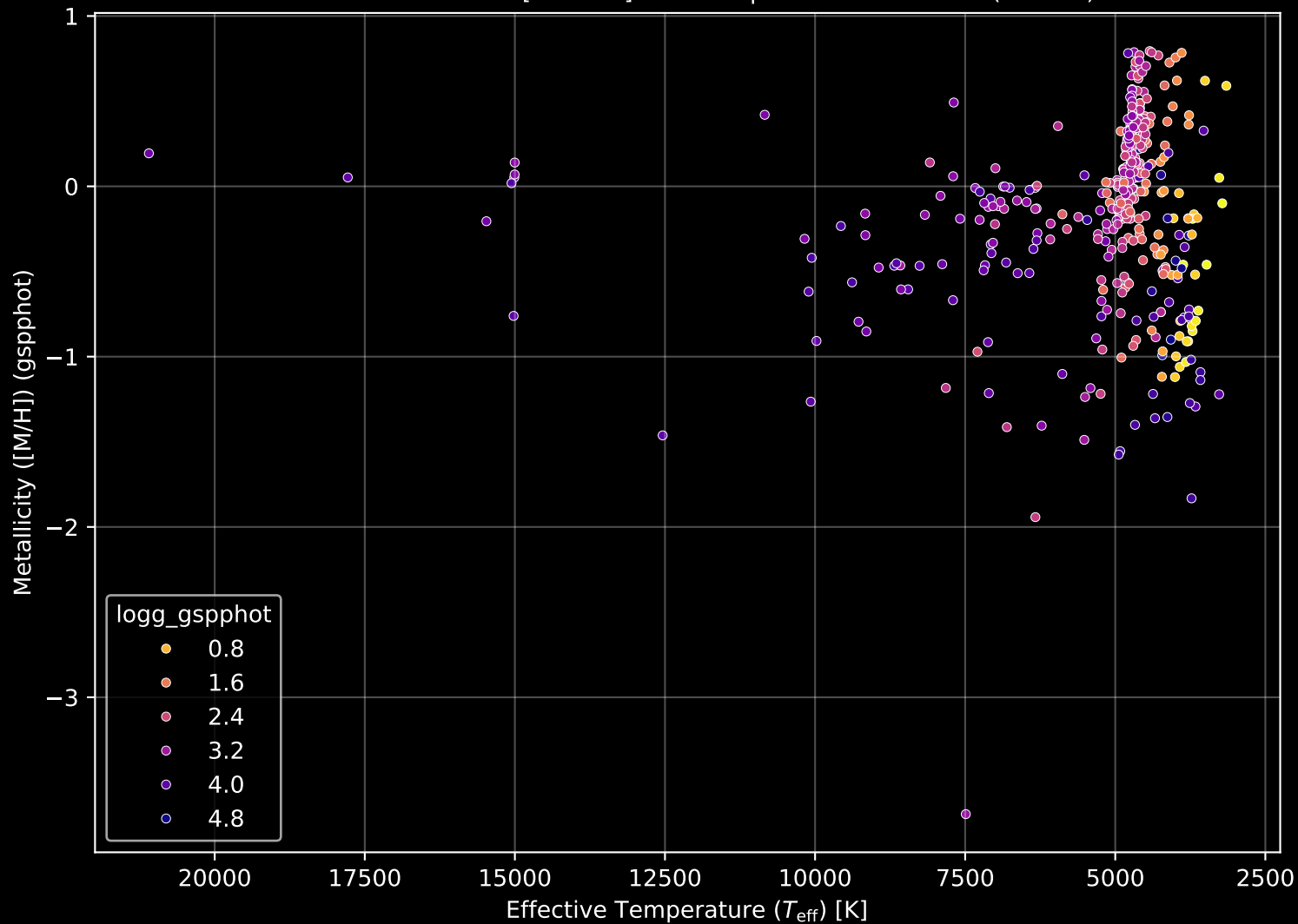
APOGEE DR17 Field: [030+00] Stellar Population Parameters (n= 396)
